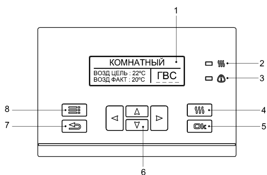
Рисунок 2. Блок управления
